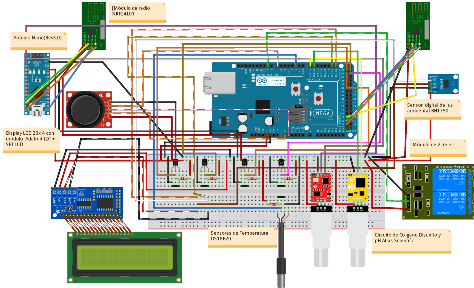
Figura 130. Diagrama general del Proyecto de Seguimiento y Control de Parámetros fisicoquímicos. Fuente: Elaboración propia desarrollado con software Fritzing versión 0.8.3.
