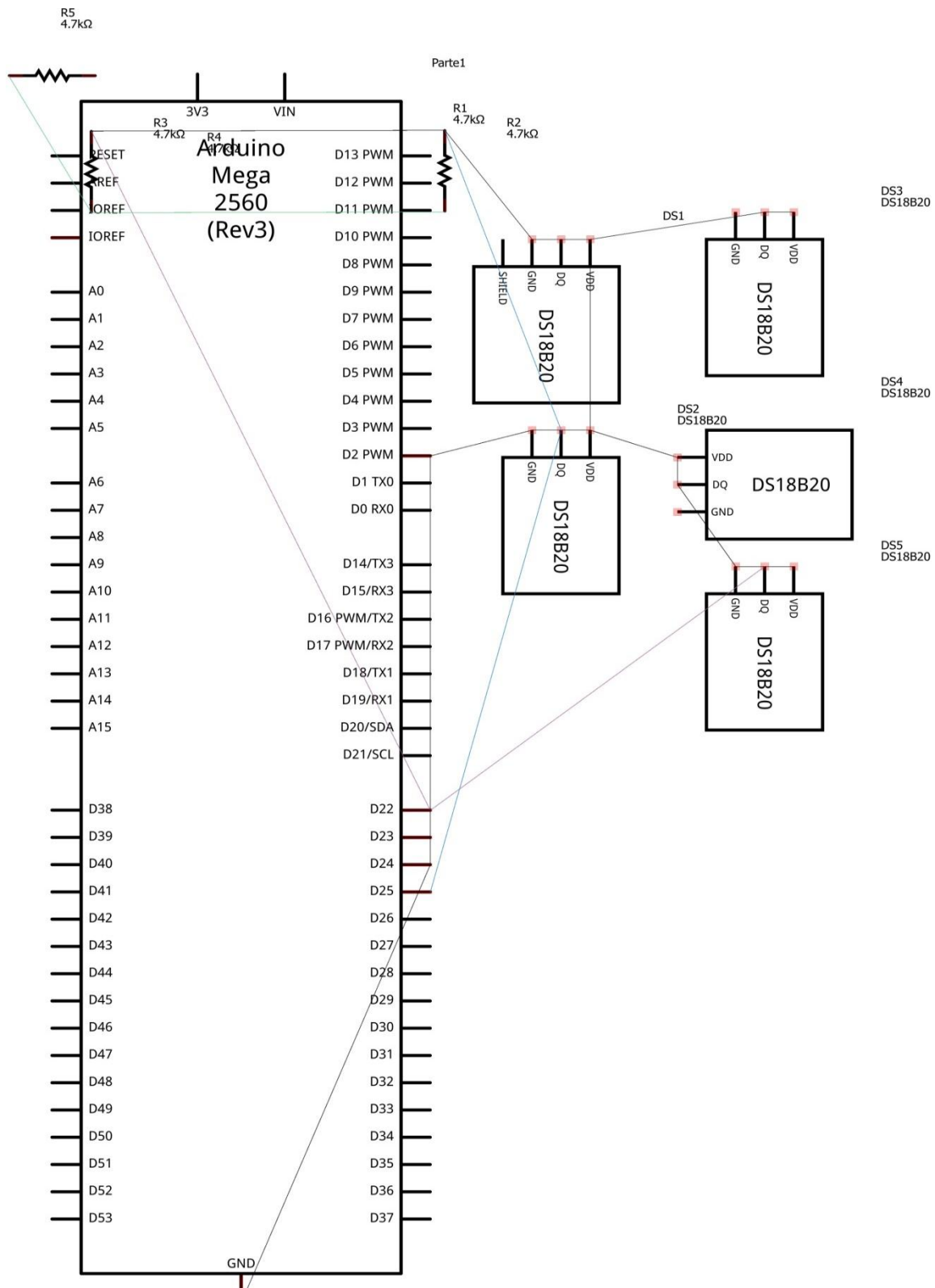
Figura 113. Diagrama de conexión de sensores con Arduino.
