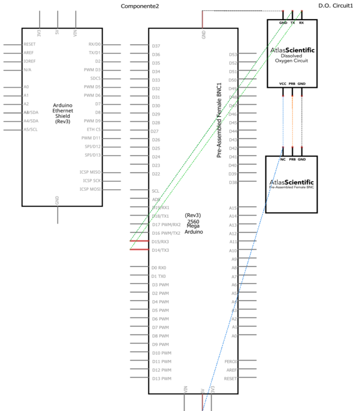
Figura 125. Diagrama esquemático con Arduino Mega 2560.
