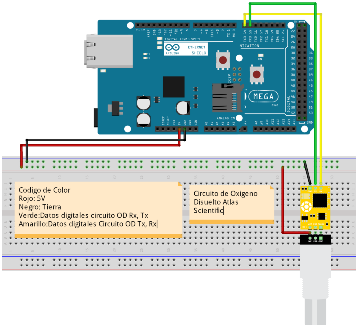
Figura 124. Sensores de Oxígeno Disuelto con Arduino Mega 2560. Fuente: Elaboración propia desarrollado con software Fritzing versión 0.8.3.
