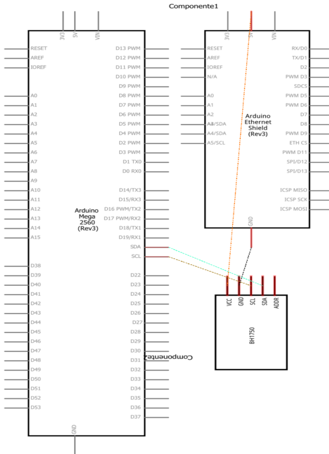
Figura 129. Diagrama de conexión entre plataforma Arduino y sensor BH1750.
